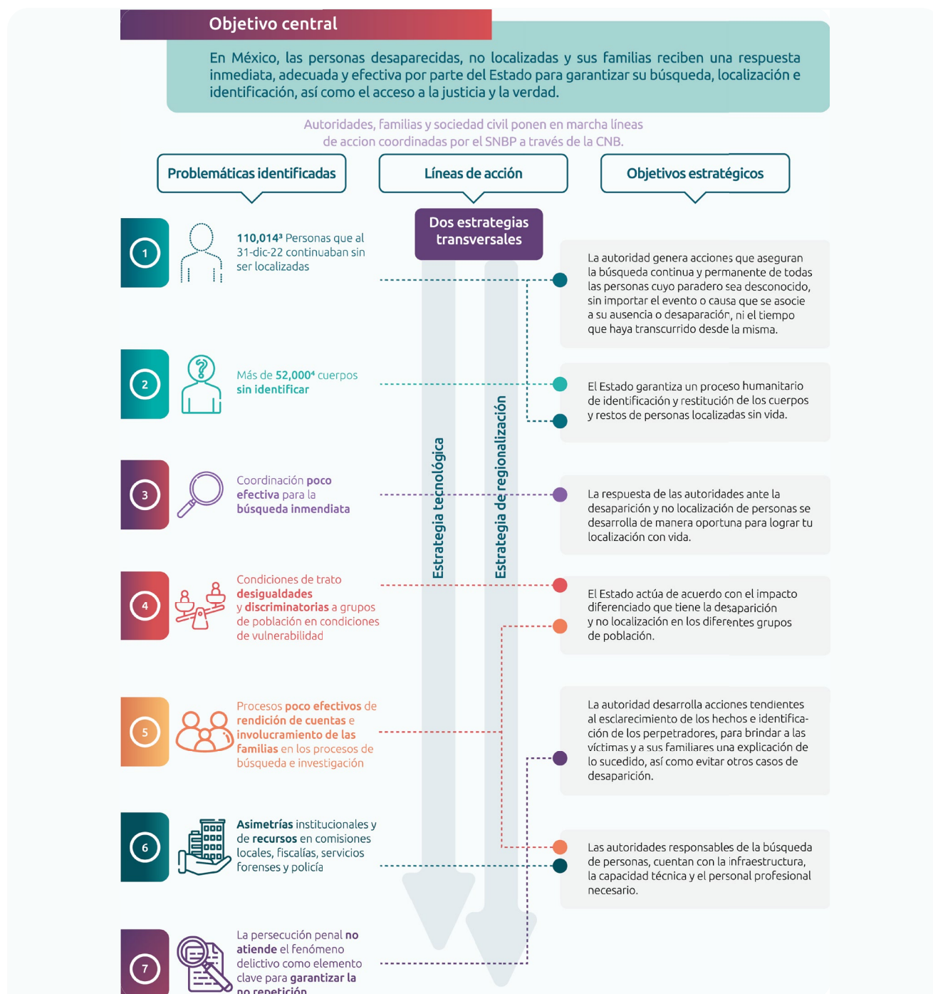
Figura 1: Causalidad programática.
